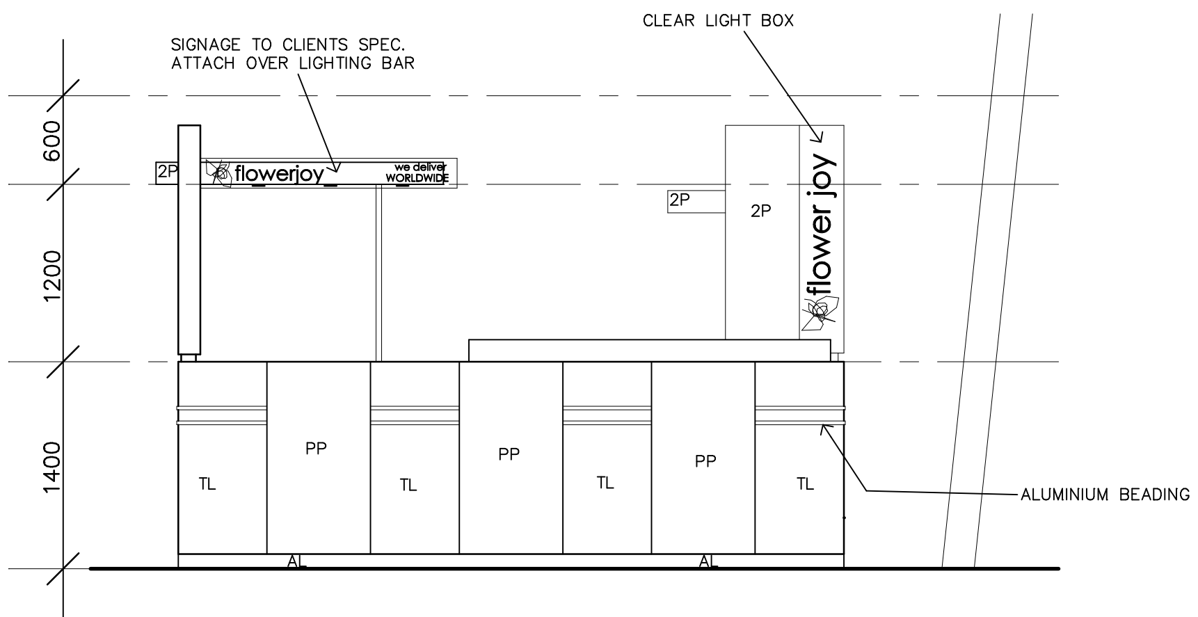
ELEVATION 3
