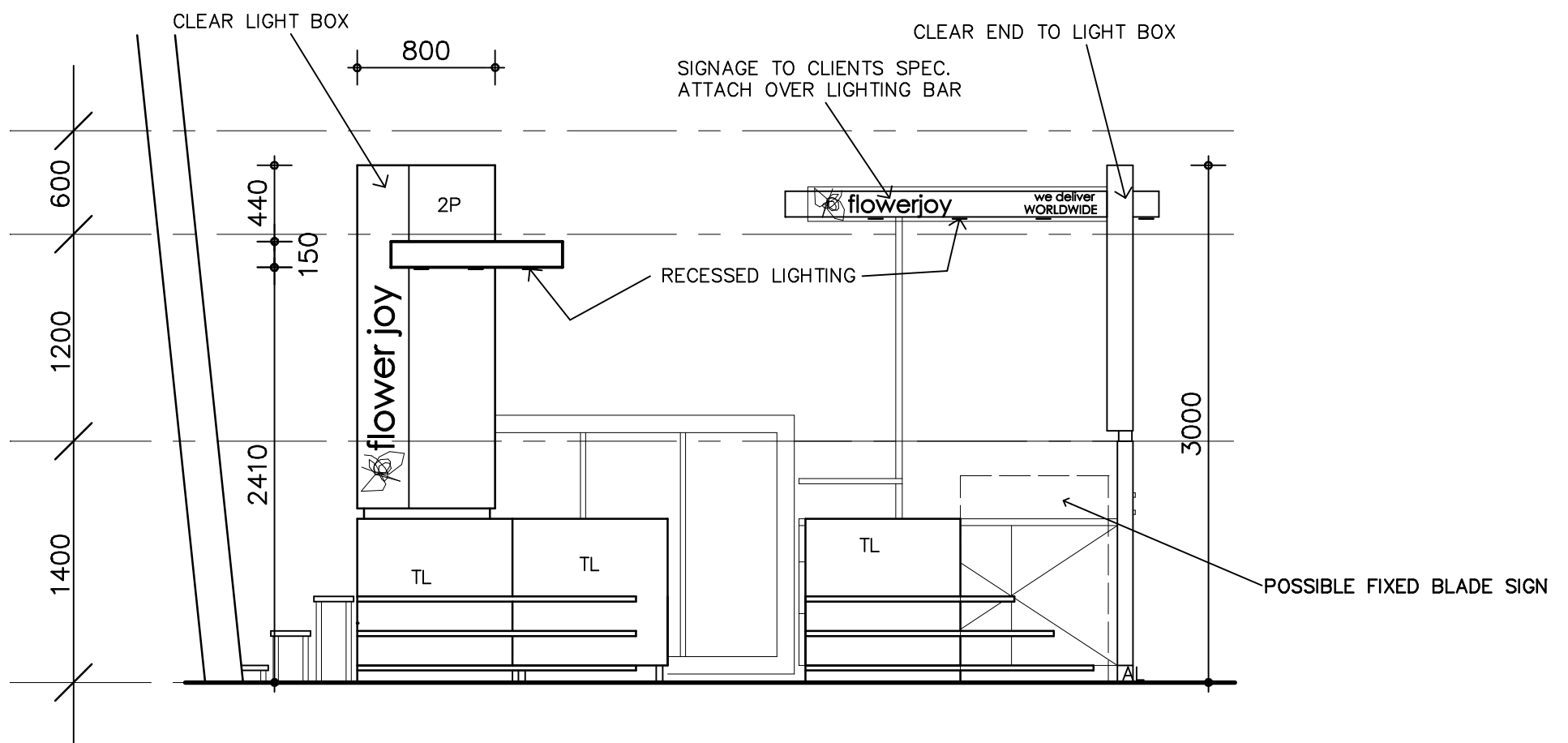
ELEVATION 1
